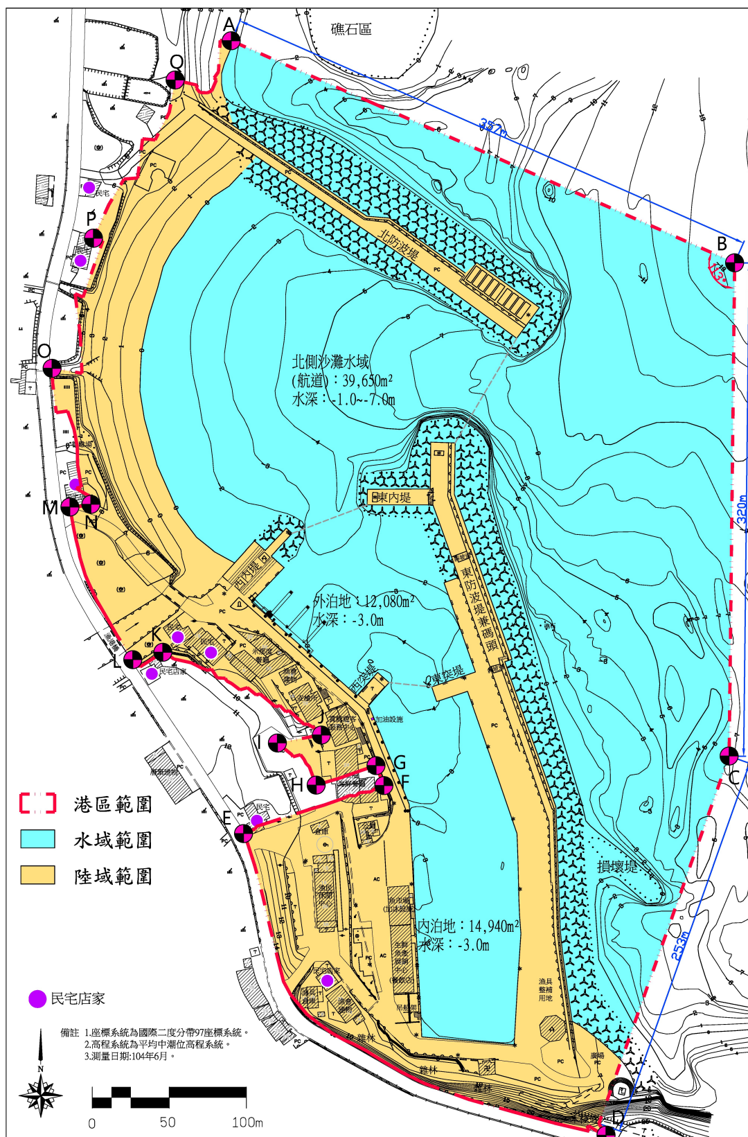
石梯漁港區域平面圖(115 年修訂版)
