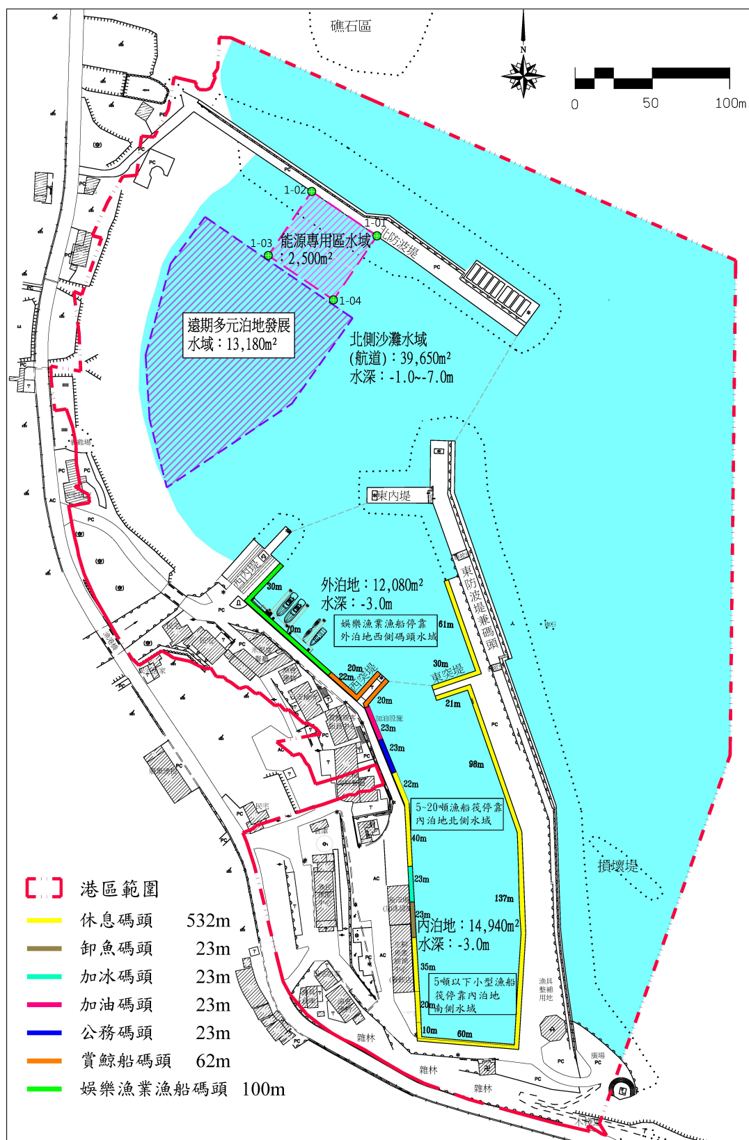
石梯漁港水域分區使用計畫圖(115 年修訂版)
