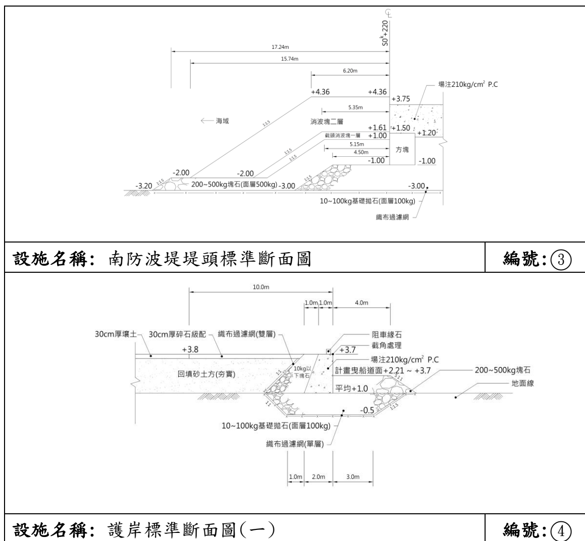
圖 8 結構標準斷面圖(續 1)
