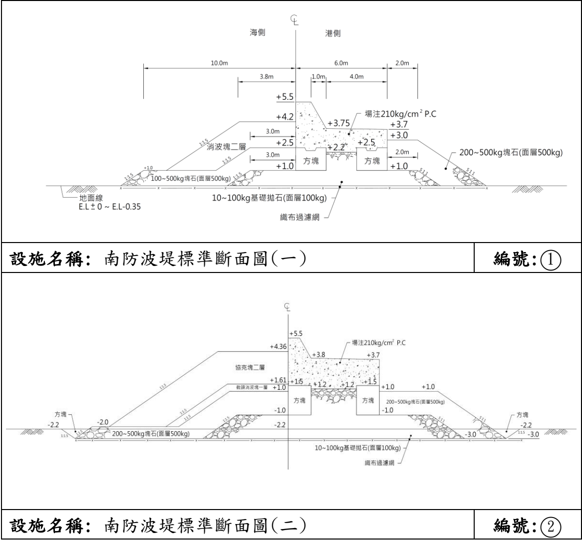
圖 6 結構標準斷面圖
