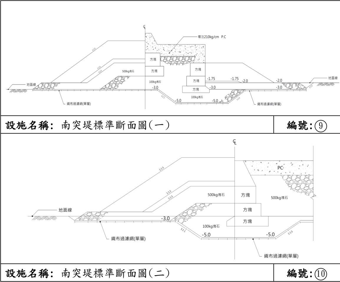
圖 14 結構標準斷面圖(續 4)
