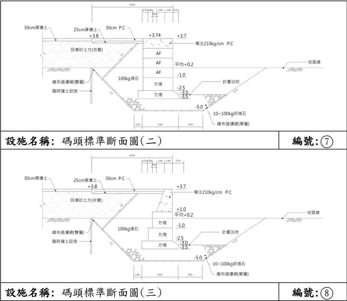
圖 12 結構標準斷面圖(續 3)
